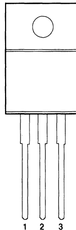
TO-220 Package (MIC2920A-xxBT)
