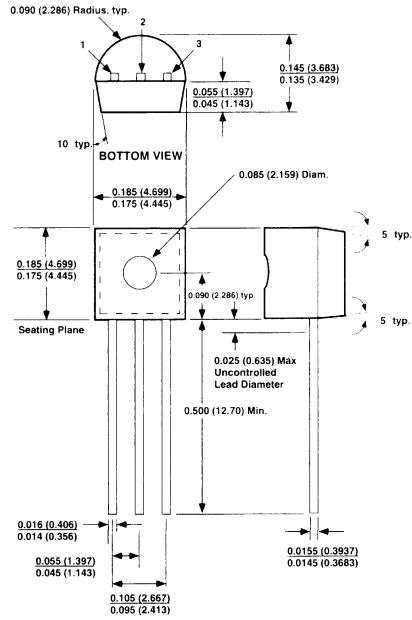
TO-92 (Z)
