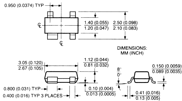
SOT-143 (M4)
