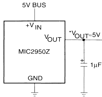
5 Volt Current Limiter
