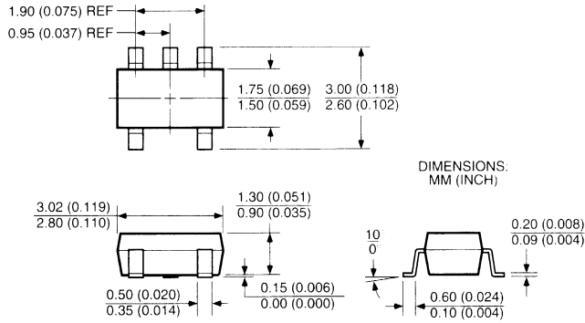
SOT-23-5 (M5)
